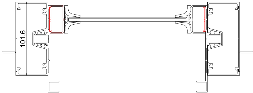
JAMB
