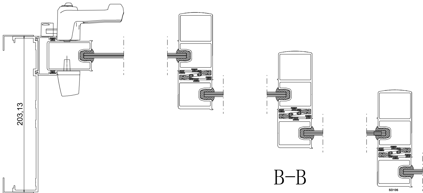
JAMB & INNERLOCK
