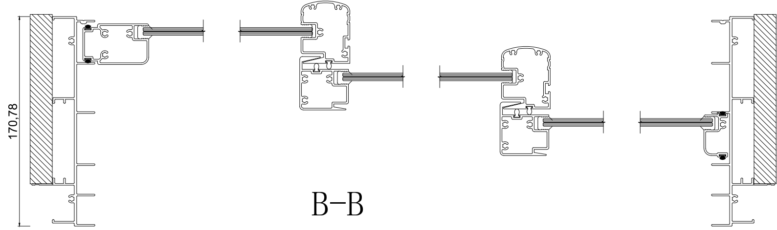
JAMB & INNERLOCK
