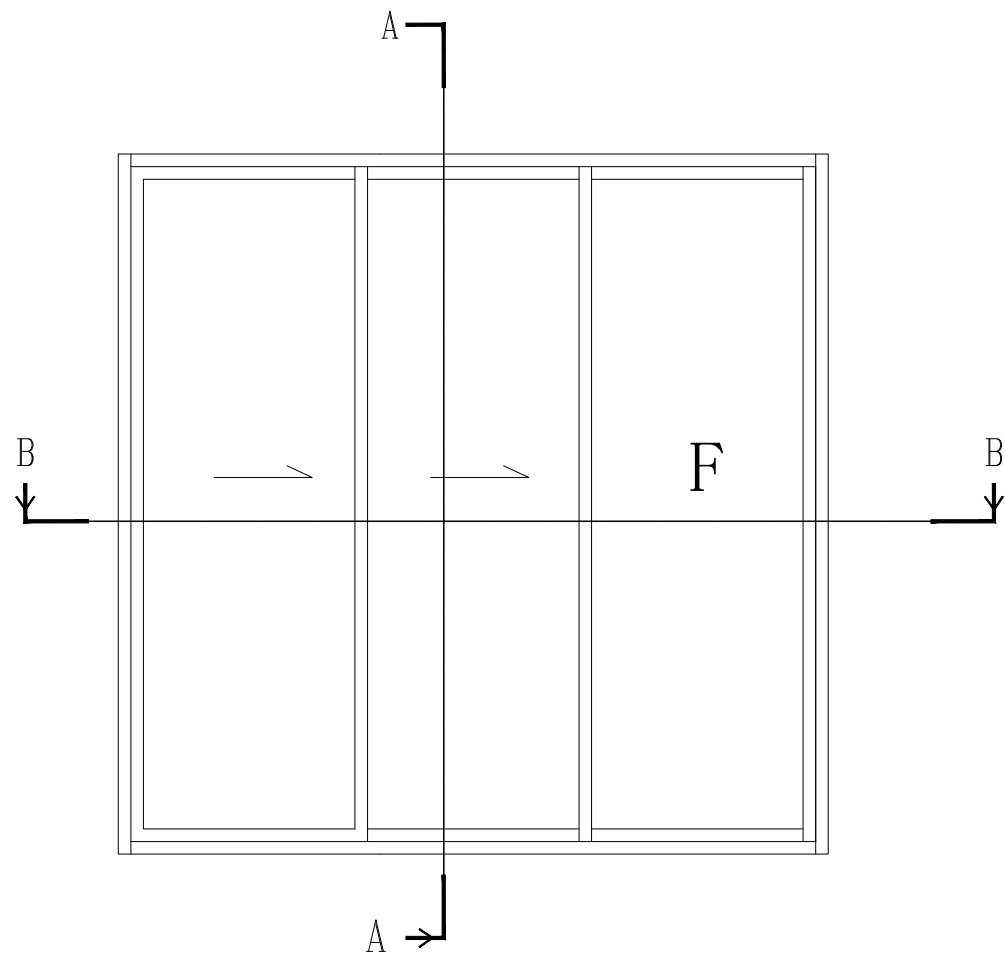
SLIDING DOOR
